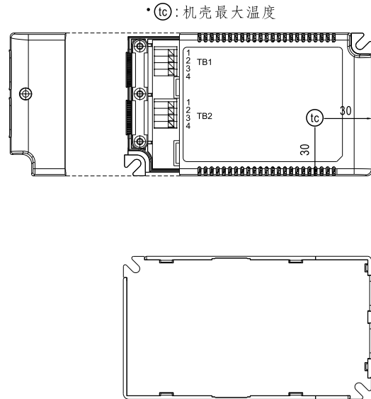
端子pin脚定义(TB2)
